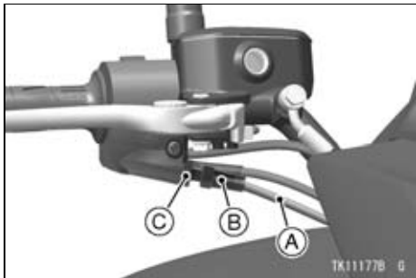
A. Cable del acelerador B. Regulador C. Contratuerca
